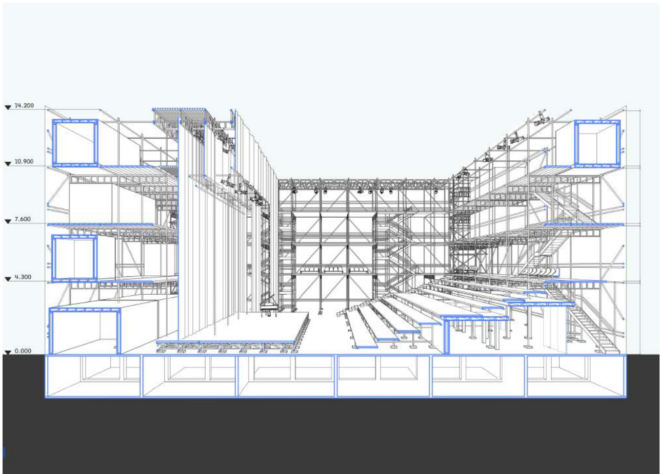
Рисунок 5.1: Перспективний розріз театру.
