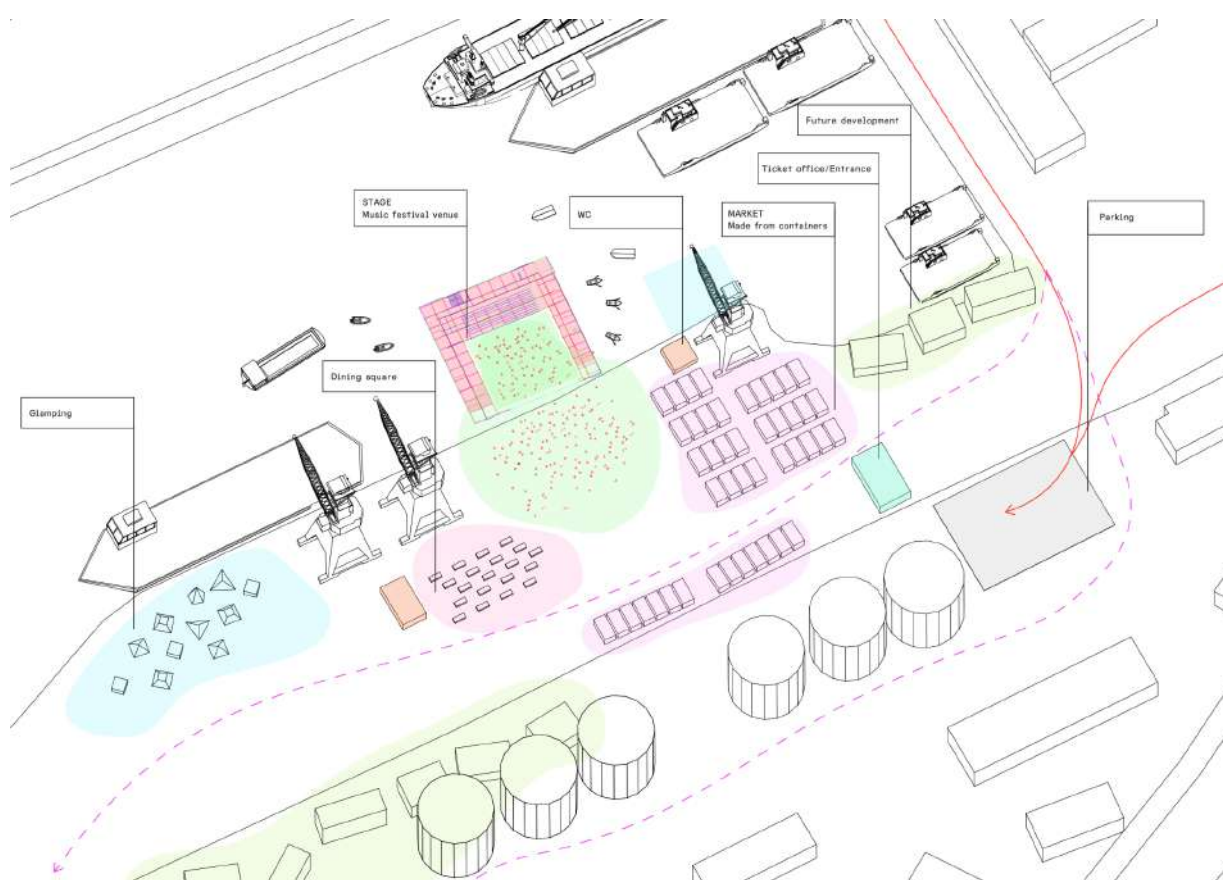
Рисунок 4.1: Зонування мастер плану.
