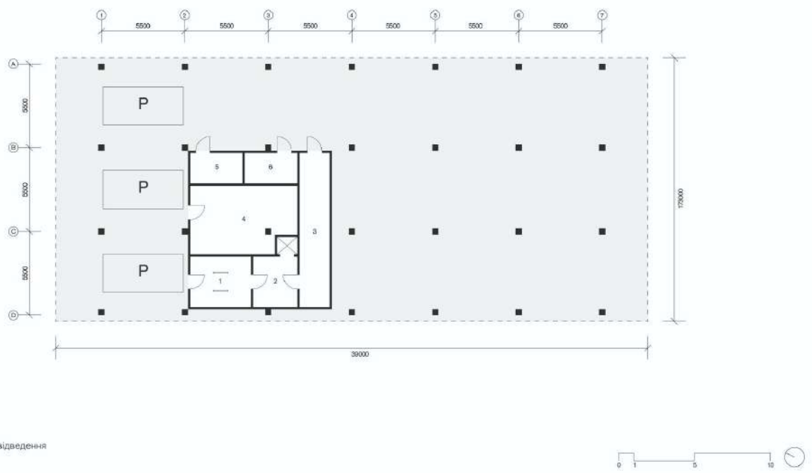
Рис. 4.2 План -1 поверху
